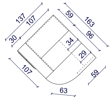
Grundriss rechter Schrank
